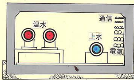
支線共同溝断面図
