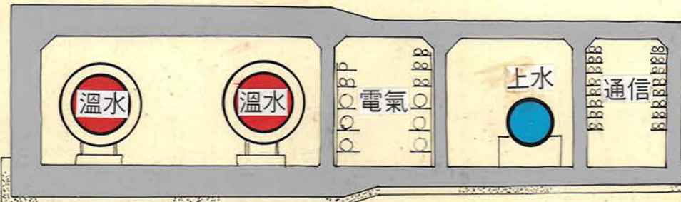
幹線共同溝断面図
